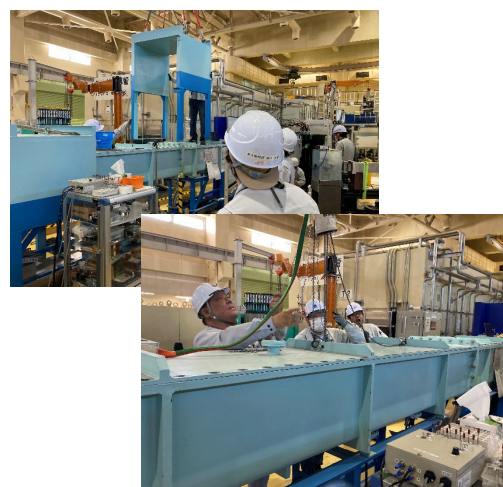
図 5, 6：SANS-U コリメータ槽解体
