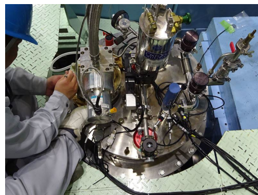
図 4：超電導電磁石（HRC）
