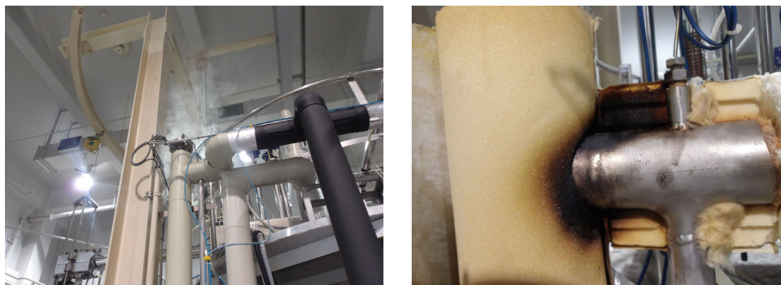
図 3. (左)トラブル発生時(発煙の様子) (右)断熱材の様子
