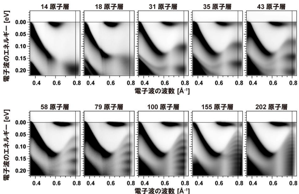
(図1) 光電子分光法で観測されたビスマス薄膜のバンド構造を、電子波のエネルギーと波数（波長の逆数）の関係で示している。黒色が信号強度の強い領域を表す。原子スケールの薄膜中における電子波の干渉が直接観測されている。
