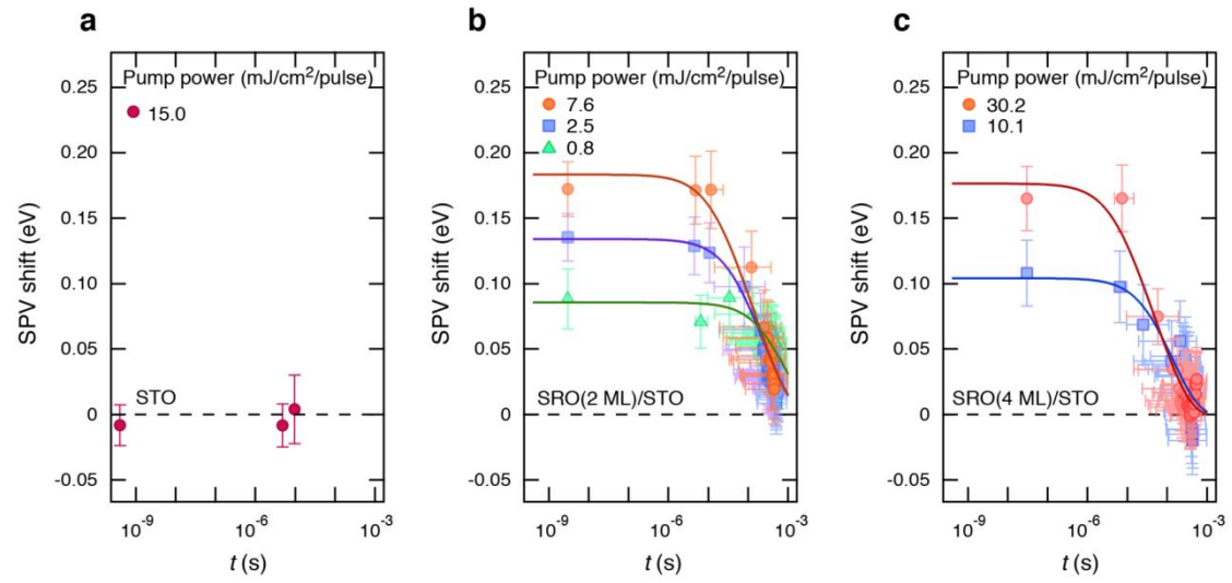
図2 \text{SrRuO}_3/\text{SrTiO}_3 (SRO/STO)ヘテロ構造の時間分解光電子分光の結果：(a) STO 基板、(b) SRO (2 層)/STO、(c) SRO (4 層)/STO。SRO 膜の存在によって t=0 で照射した紫外線パルス光に対して光起電力 (SPV shift) が発生し、時間とともに緩和していく様子が分かる。
